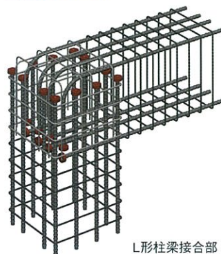
L形柱梁接合部
