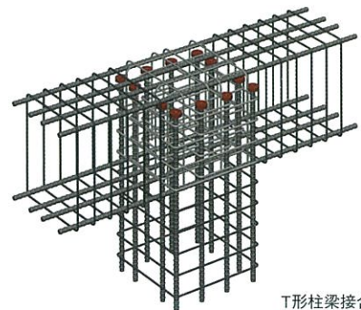
T形柱梁接合部
